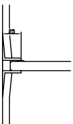
Rejtett lábazati profil
