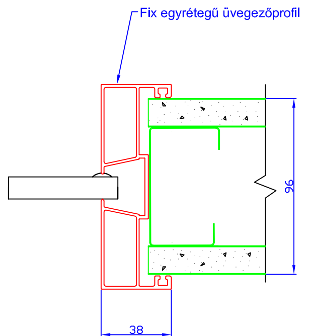
Egyrétegű üvegezés kerettel gipszkartonfalhoz csatlakozó profil
