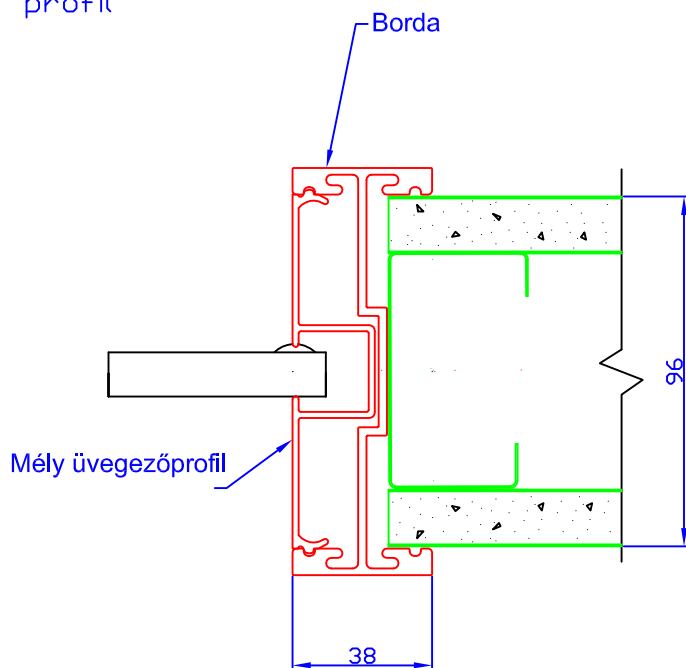
Egyrétegű üvegezés kerettel gipszkartonfalhoz csatlakozó profil
