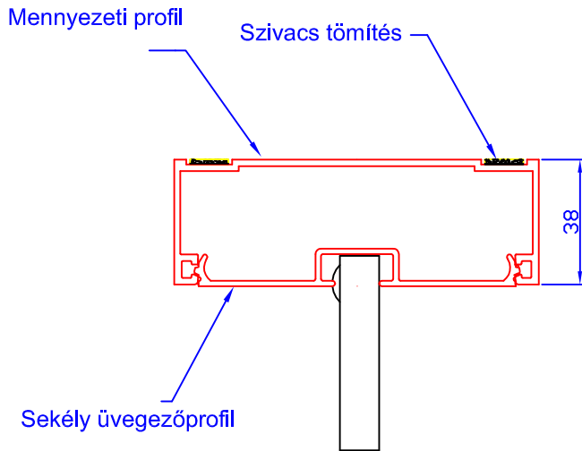
Egyrétegű üvegezés kerettel Mennyezeti profil
