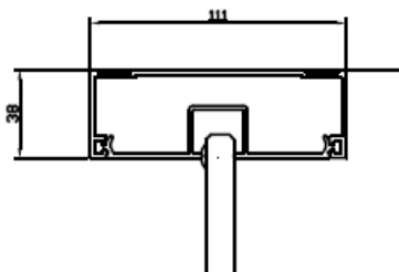
Mennyezeti profil
