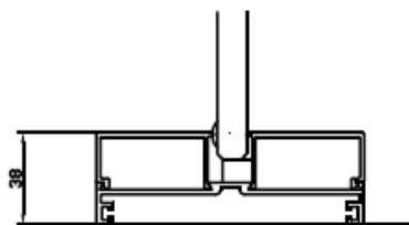
Lábazati profil
