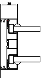
Lábazati profil
