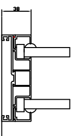
Lábazati profil
