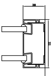
Födém lehajlását toleráló mennyezeti profil
