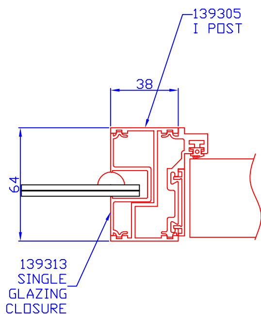
Ajtók és egyrétegű üvegezés találkozása
