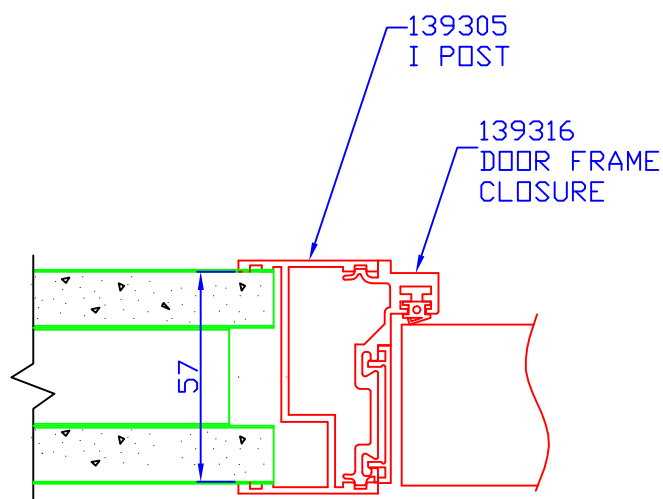
Ajtók és gipszkartonfal találkozása
