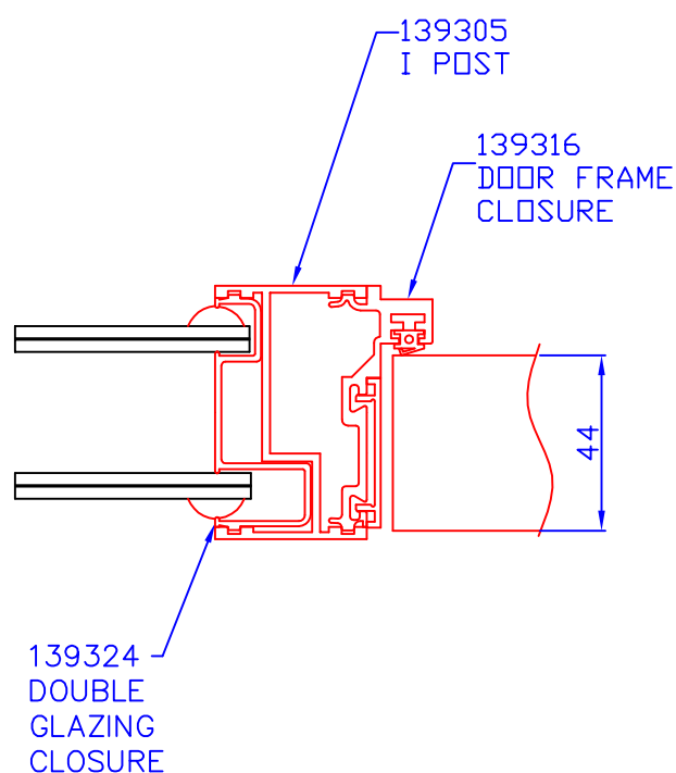
Ajtók és kétrétegű üvegezés találkozása
