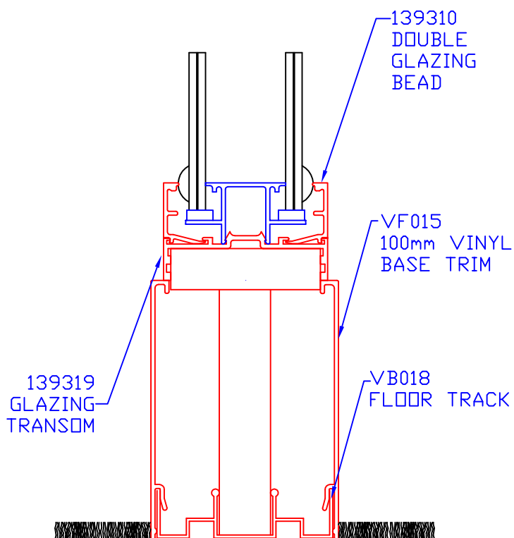
Kétrétegű üvegezés – magas lábazati profil
