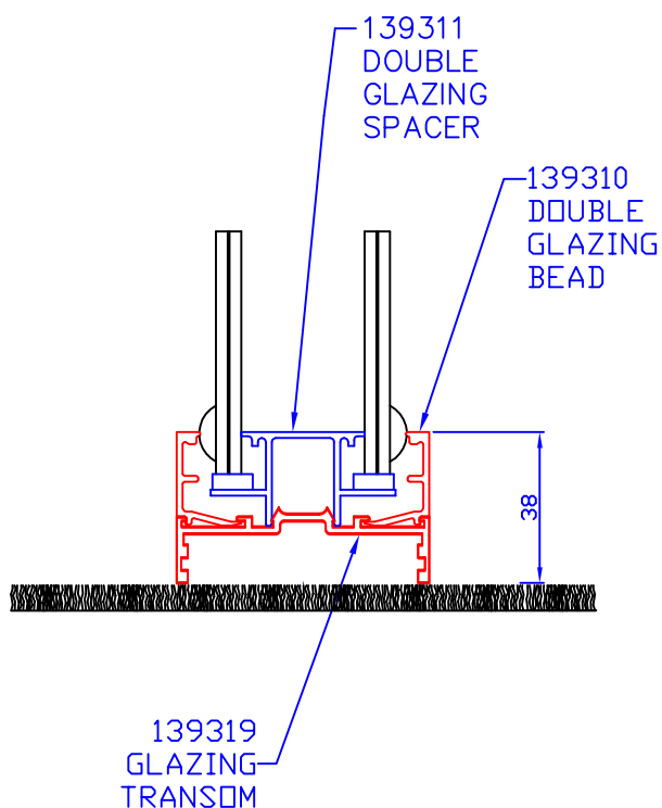
Kétrétegű üvegezés – lábazati profil
