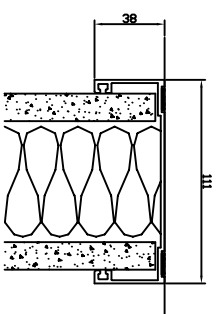
Mennyezeti profil
