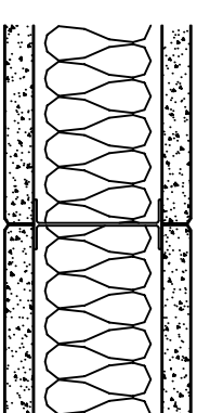
Függőleges toldás
