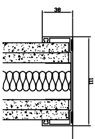
Mennyezeti profil
