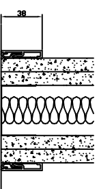
Lábazat
