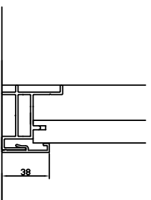
Lábazat
